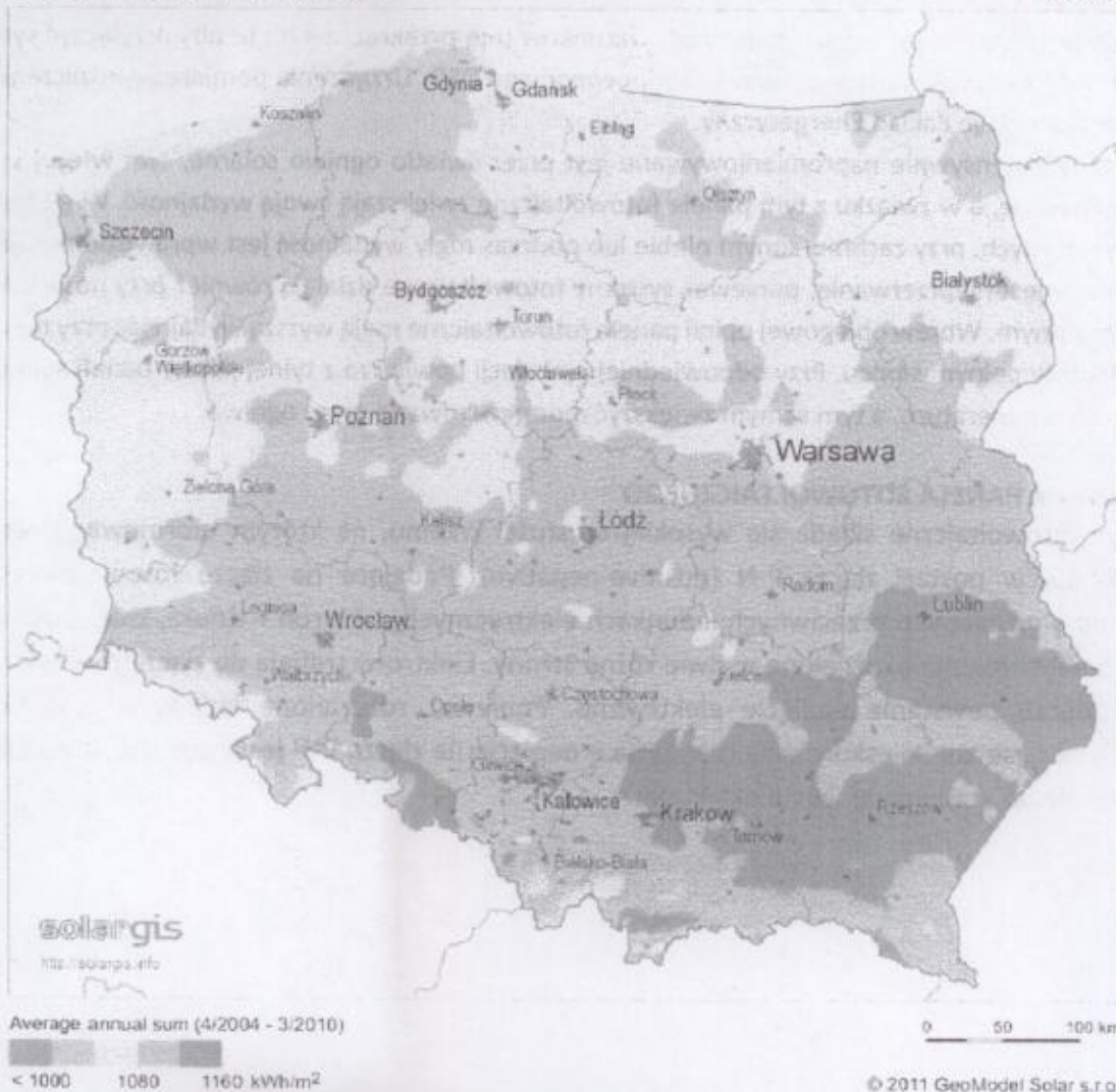
Rysunek 2 Rozkład promieniowania słonecznego na terenie Polski
