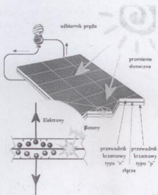
Rysunek 3 Zasada działania panelu
