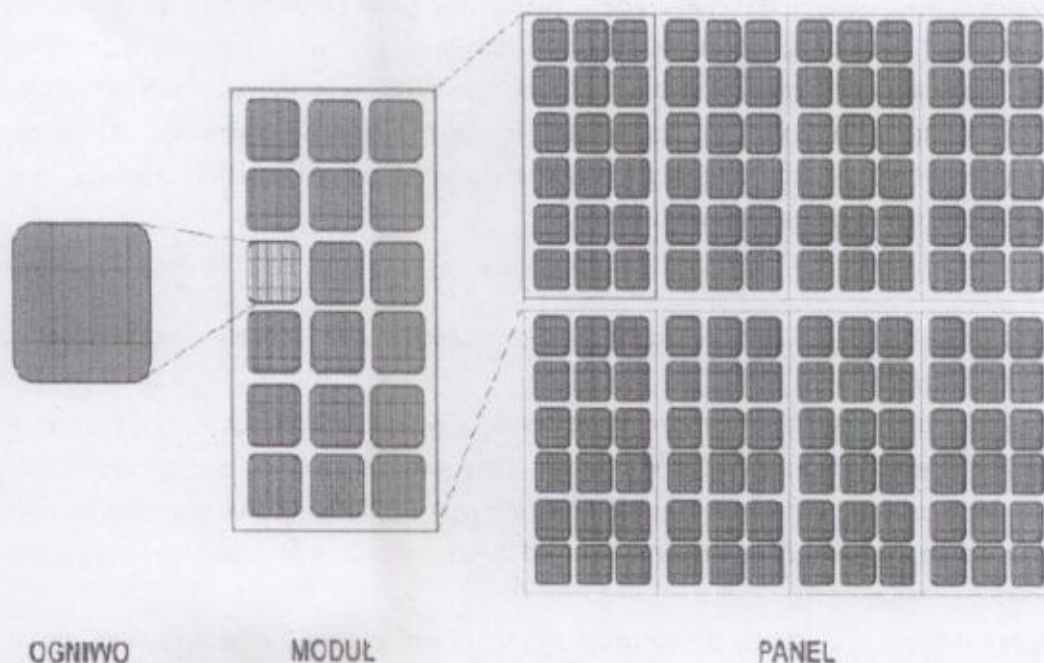
Rysunek 4 Budowa panelu
