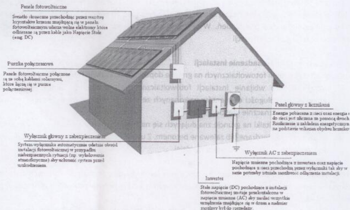
Rysunek 6 Sposób podłączenia instalacji do sieci
